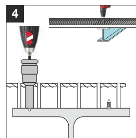
4 S-BT Bolzen in das Bohrloch einschrauben.
