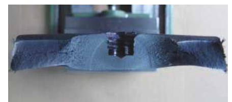
Bruchfläche
