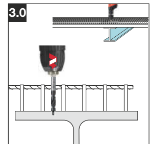
3.0 Mit dem Stufenbohrer TS-BT vorbohren.
