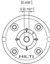
Gitterrostbefestigungsscheibe X-FCM-R
