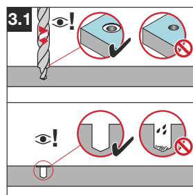
3.1 Bohren, bis die Stufe einen Glanzring erzeugt. Das Bohrloch und der umliegende Bereich müssen sauber, trocken und rückstandsfrei sein.
