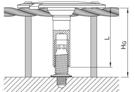
Gitterrostbefestigungsscheibe X-FCM-R
