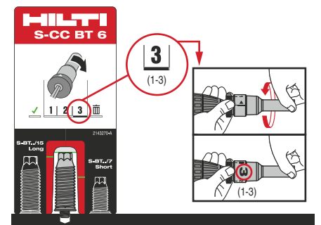
Aufbau und Funktion der Prüfschablone S-CC BT
